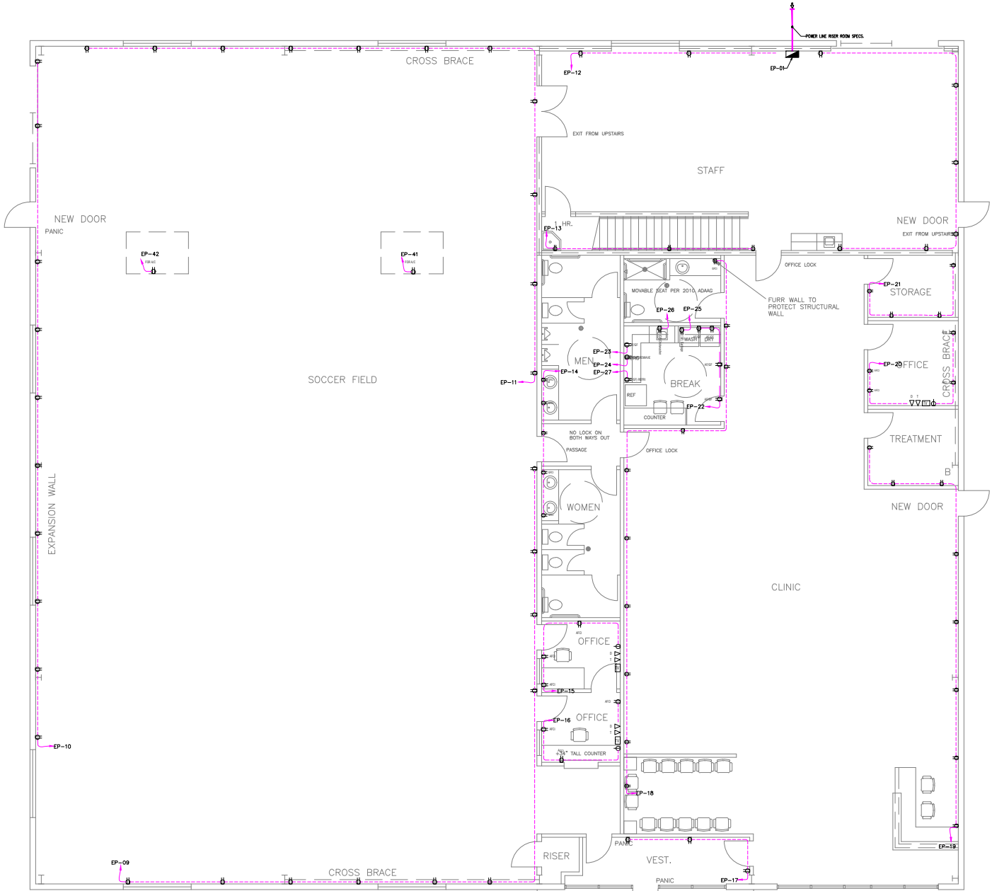
EL 03 SCALE 1/16"=1'-0"
